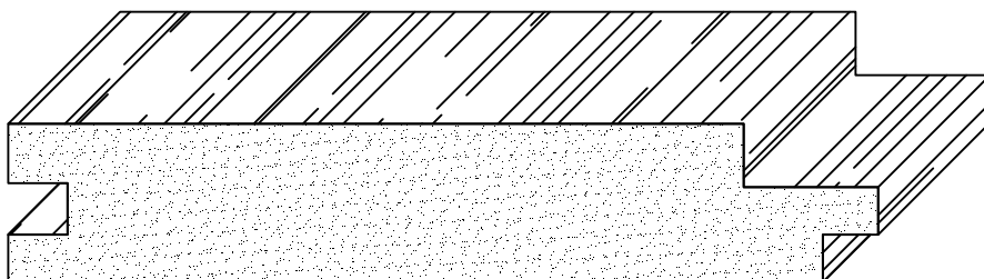
Canteria 1x5 avance 103mm codigo 3121
