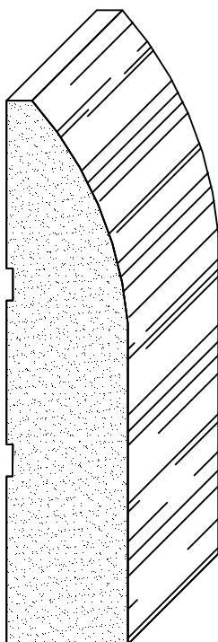
guardapolvo 1x4 20x85 mm Codigo 3035
