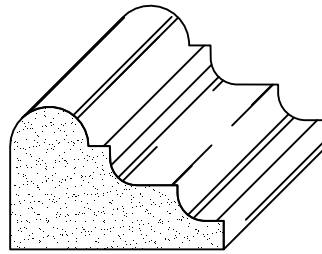
collerin 1E 20x30mm codigo 2701
