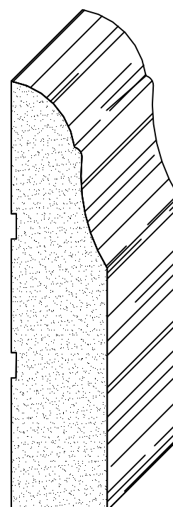
guardapolvo 1x4 20x85 mm Codigo 3033
