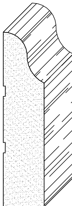
guardapolvo 1x4 20x85 mm Codigo 3036
